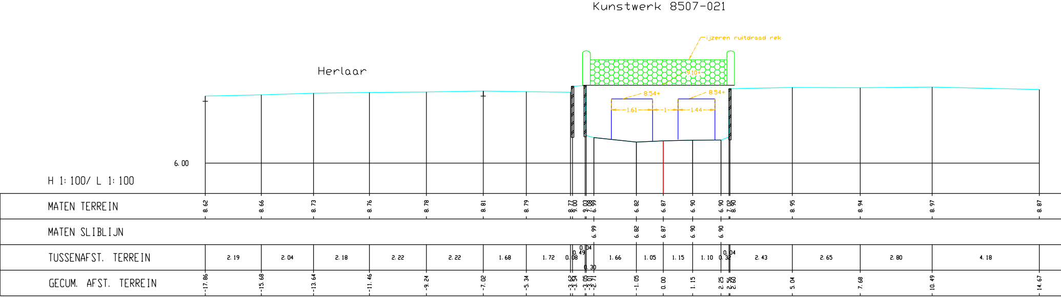
Wimp, Dwarsprofiel 026
