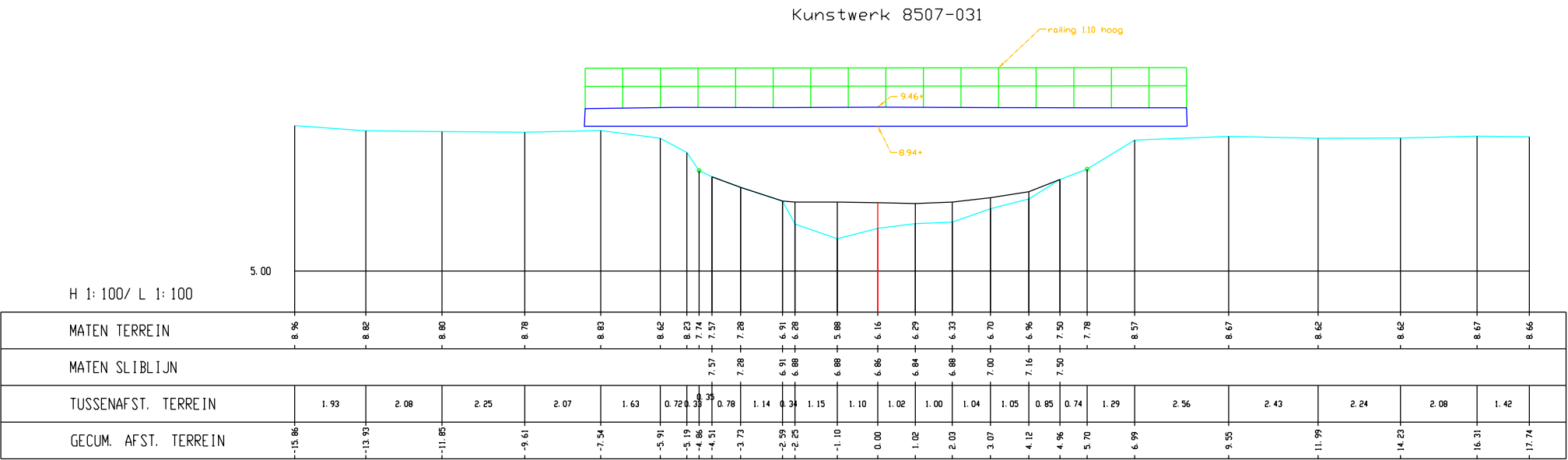
Wimp, Dwarsprofiel 049
