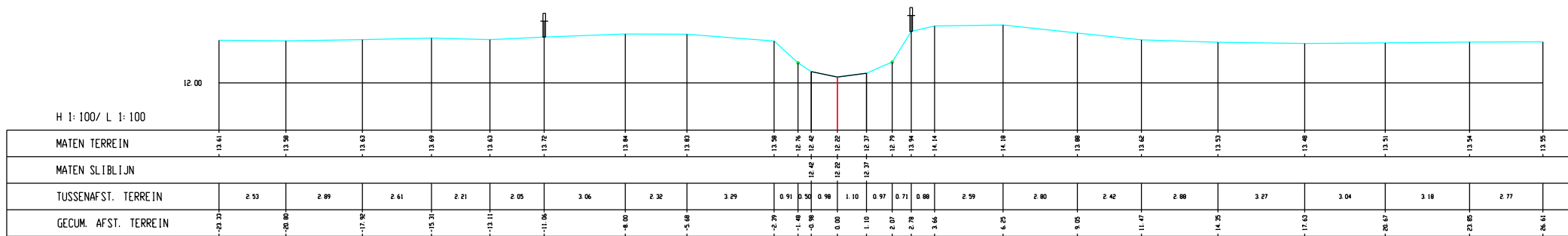
Winge, Dwarsprofiel 138
