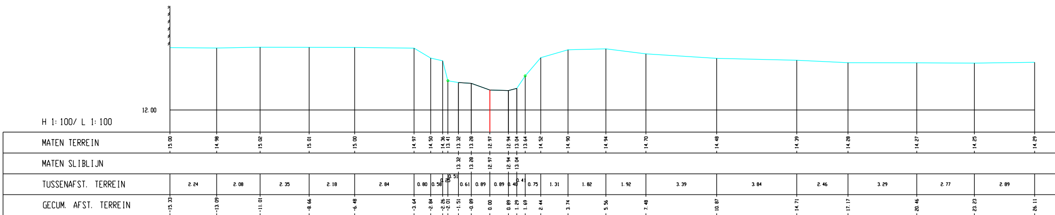
Winge, Dwarsprofiel 176
