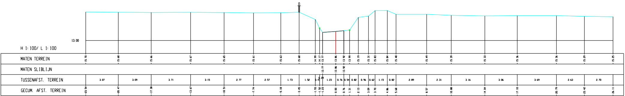
Vinge, Dwarsprofiel 211
