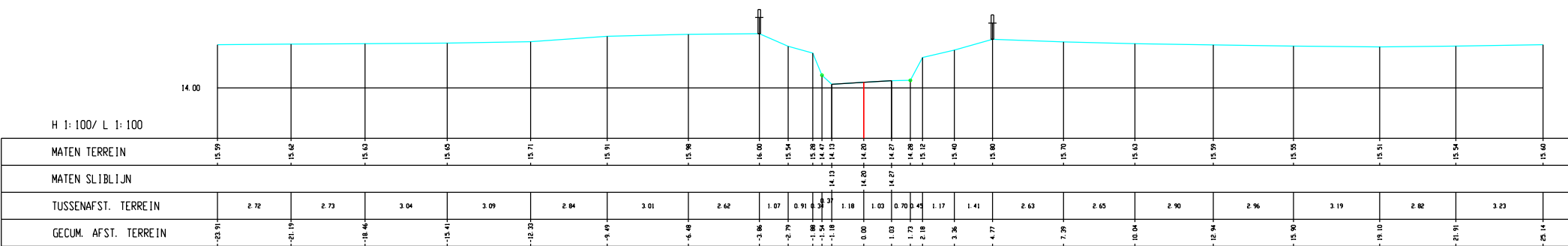
Winge, Dwarsprofiel 214
