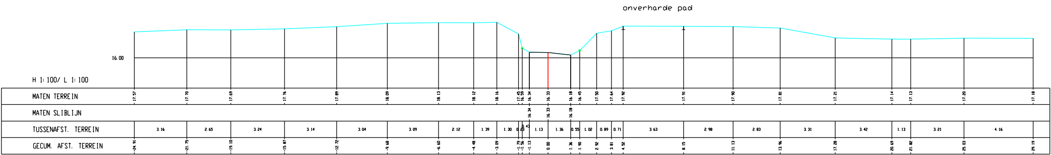
Winge, Dwarsprofiel 245
