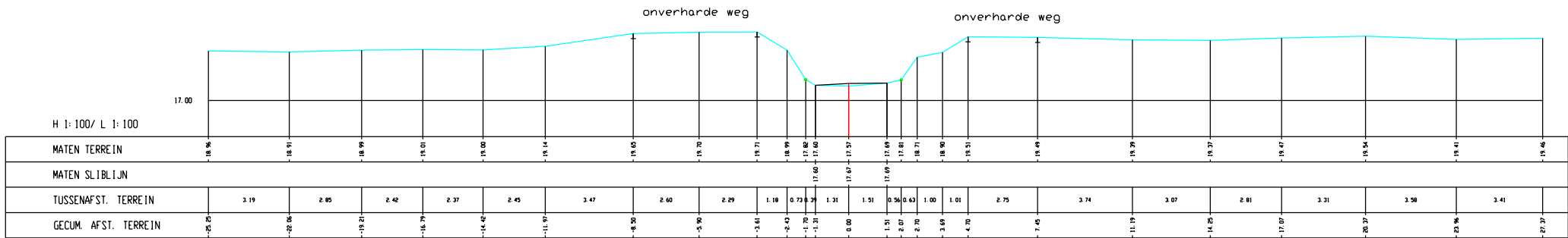
Winge, Dwarsprofiel 276
