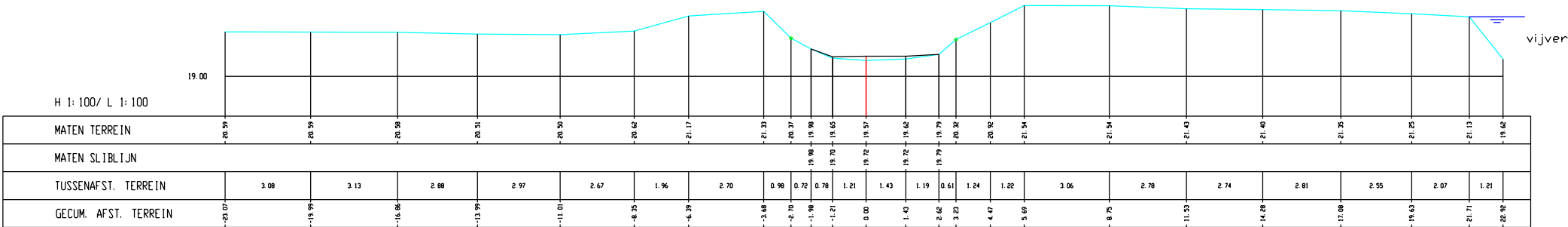
Winge, Dwarsprofiel 290
