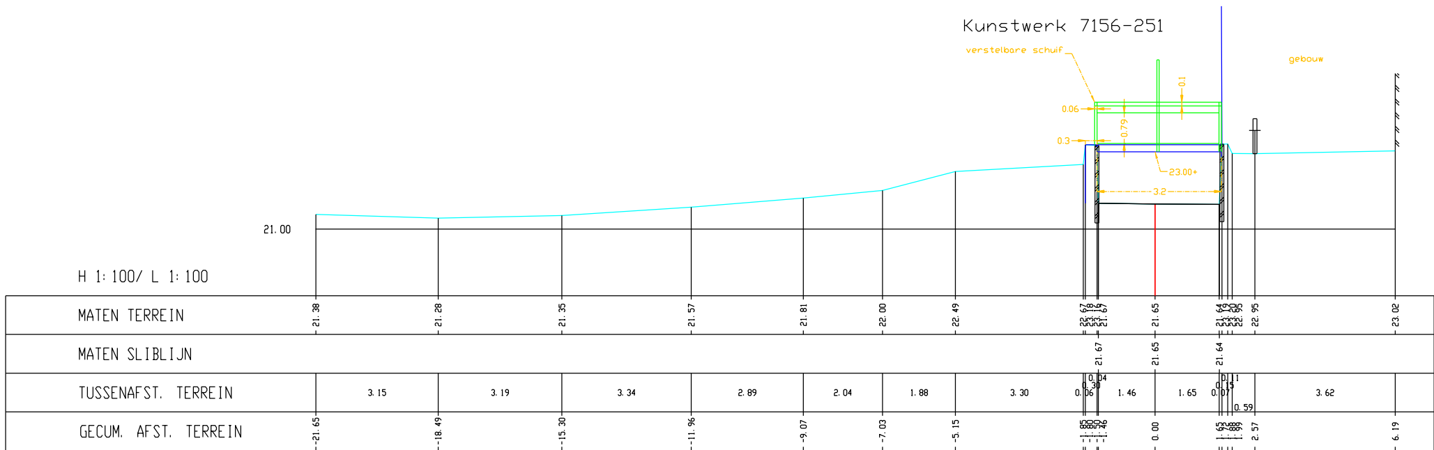
Winge, Dwarsprofiel 300
