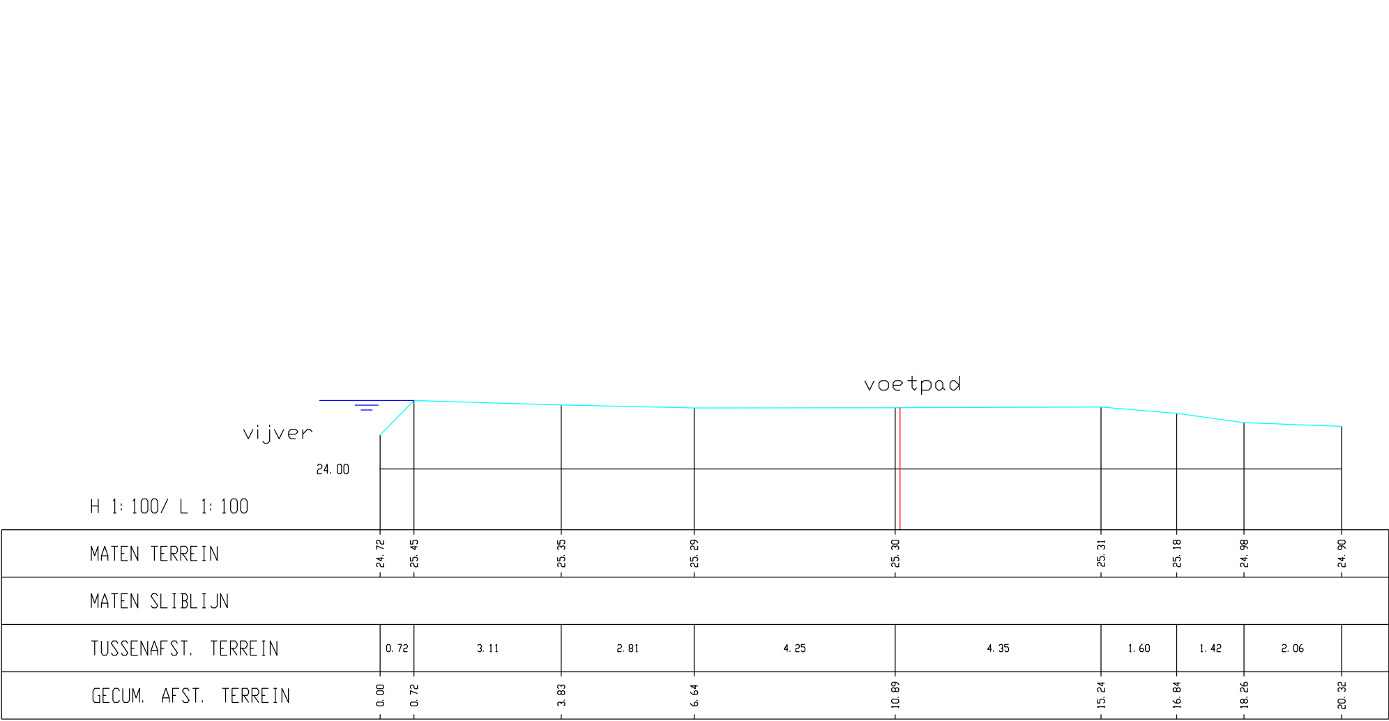
Winge, Dwarsprofiel 334
