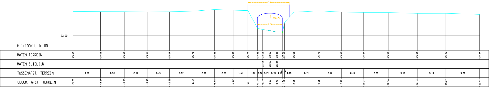
Winge, Dwarsprofiel 340
