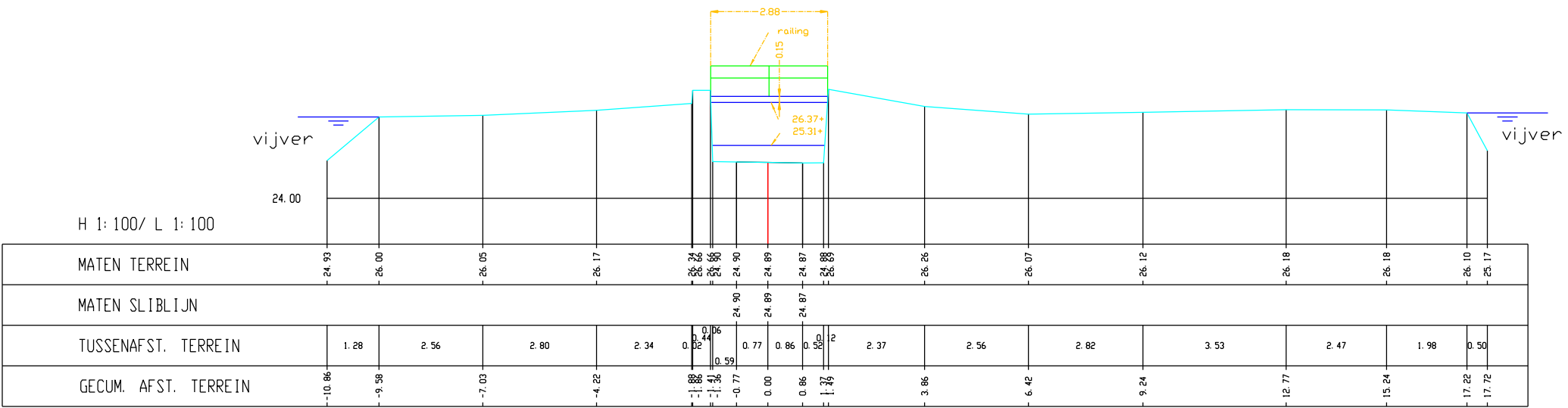
Winge, Dwarsprofiel 344
