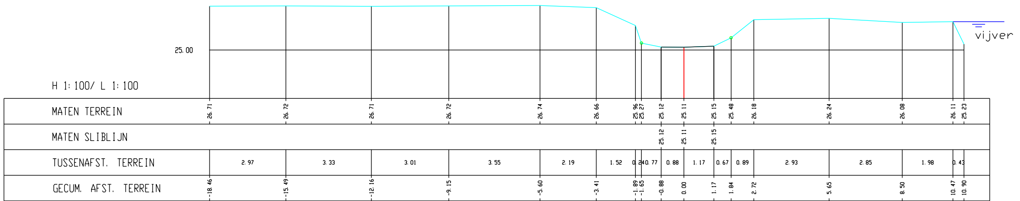
Winge, Dwarsprofiel 347
