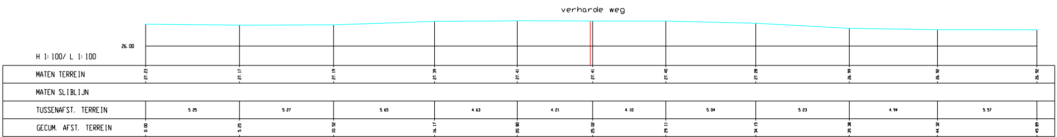
Winge, Dwarsprofiel 357
