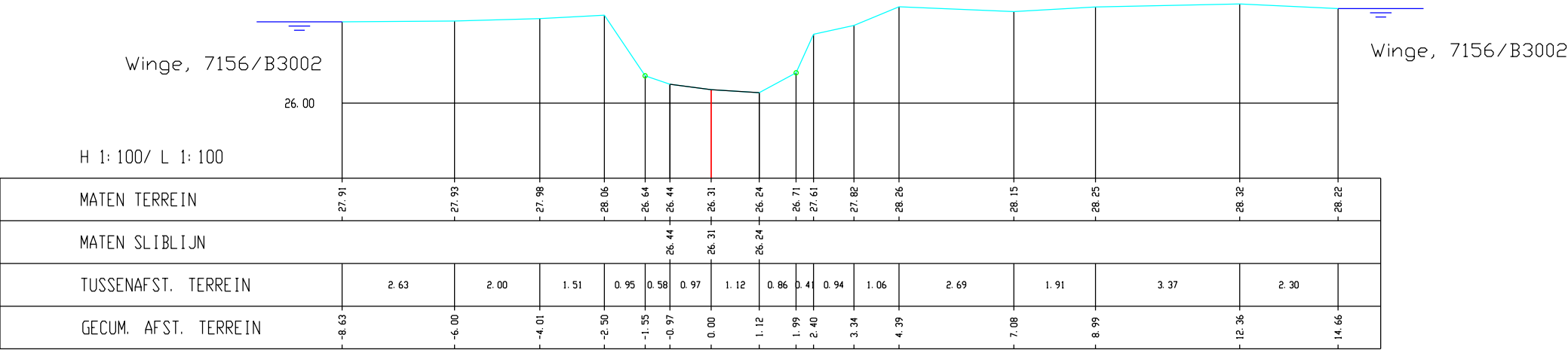
Winge, Dwarsprofiel 374
