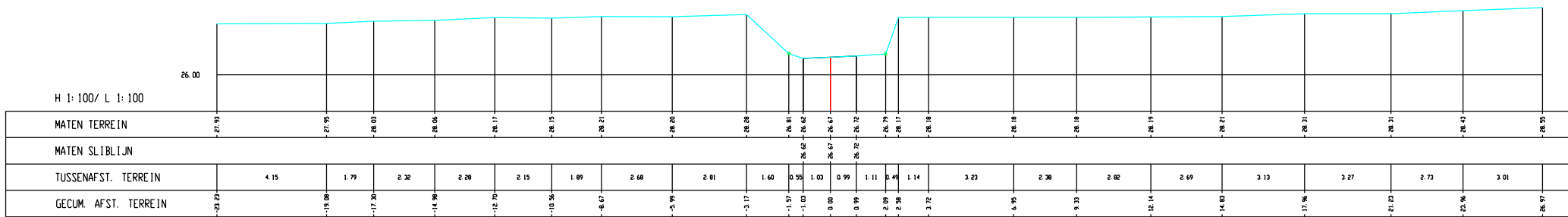
Winge, Dwarsprofiel 380
