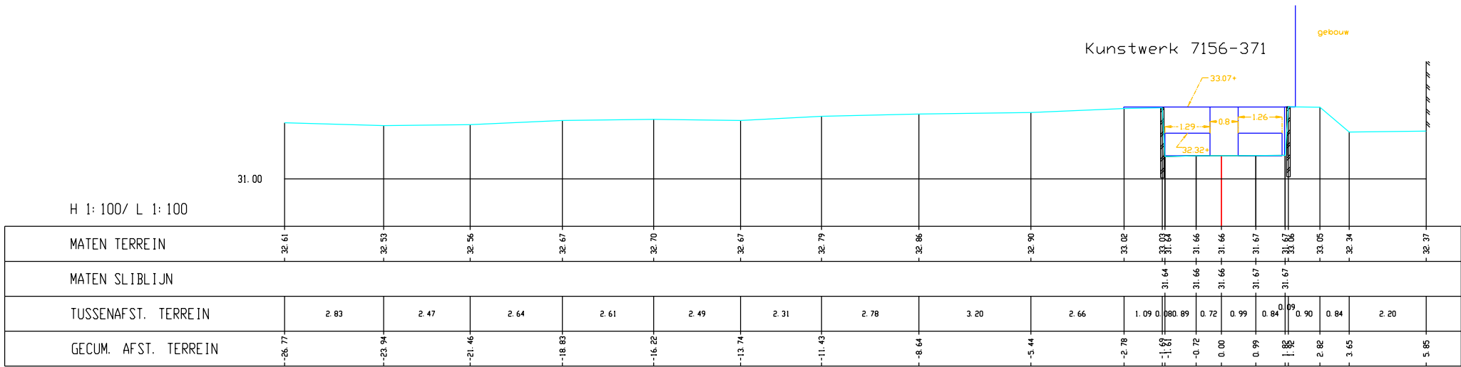
Winge, Dwarsprofiel 409
