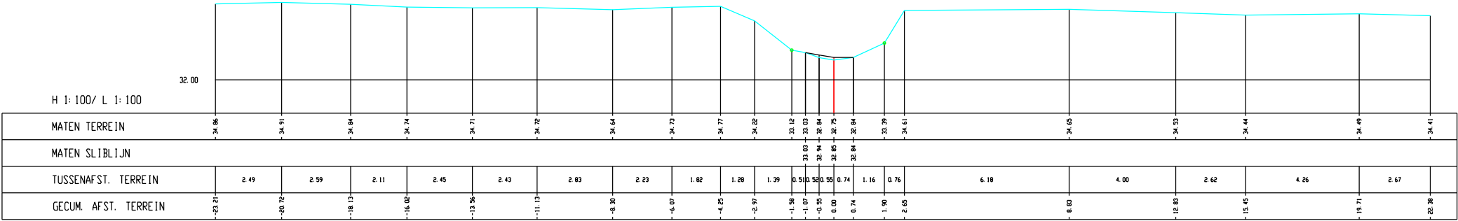
Winge, Dwarsprofiel 441
