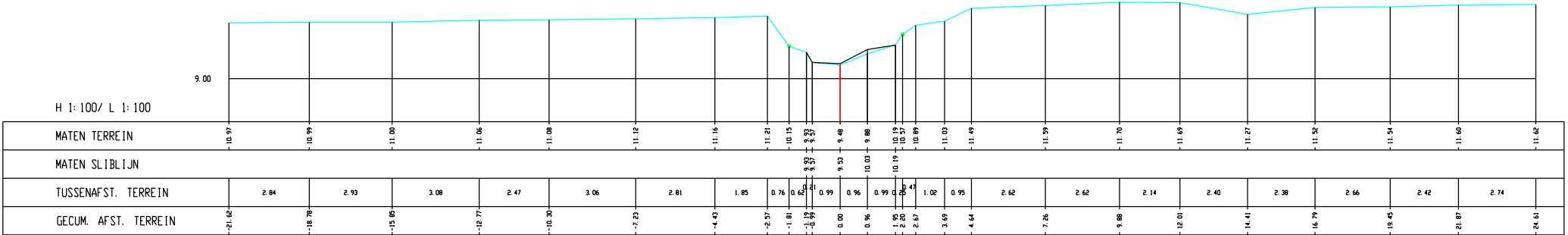
Winge, Dwarsprofiel 046
