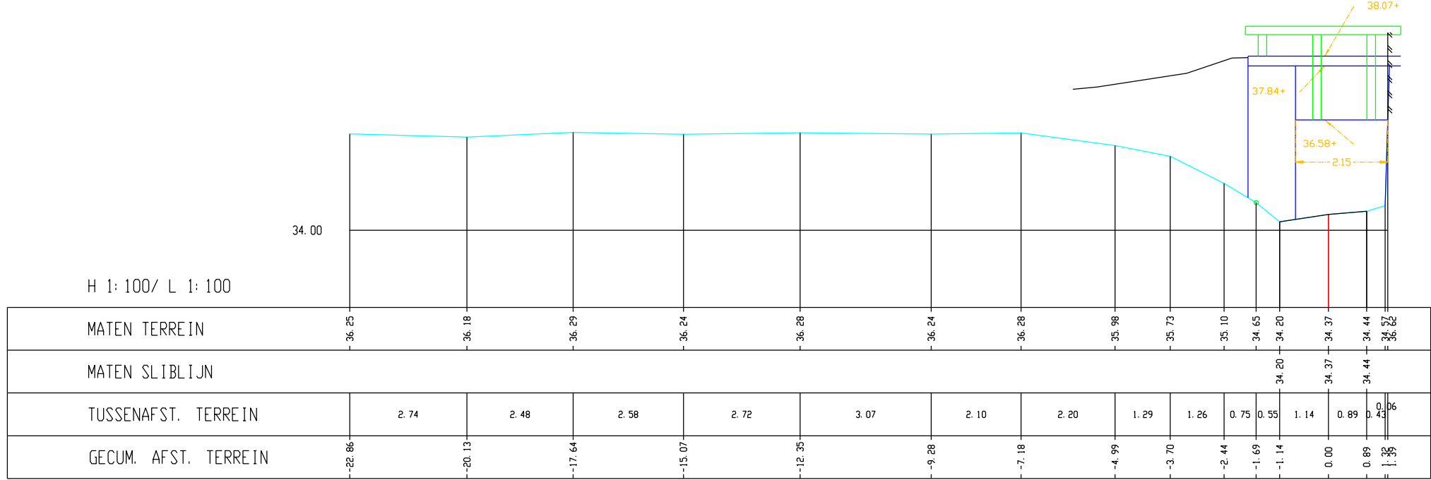
Winge, Dwarsprofiel 460
