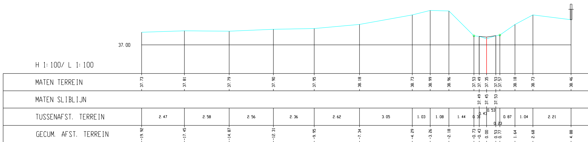
Winge, Dwarsprofiel 475
