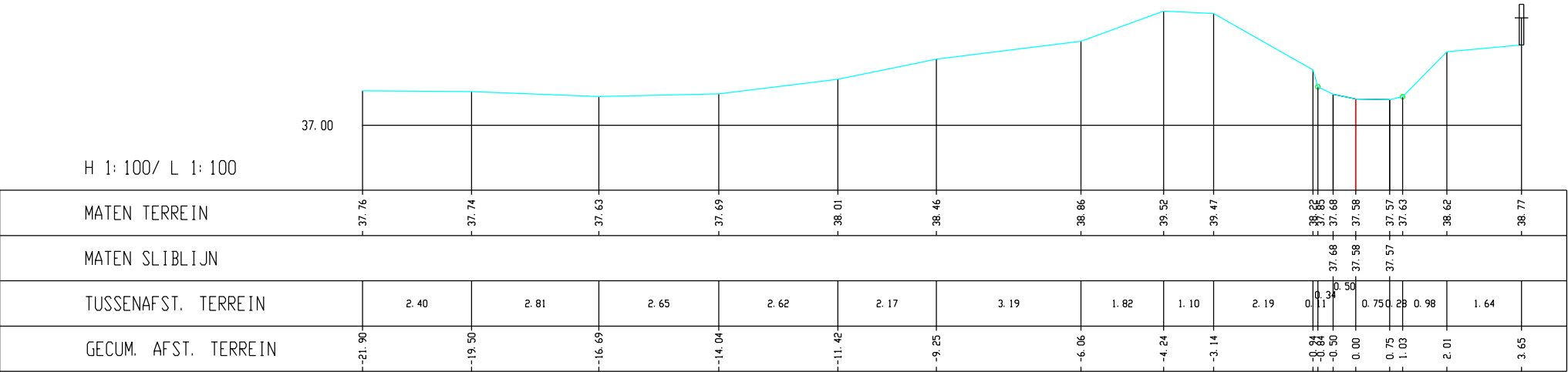
Winge, Dwarsprofiel 476
