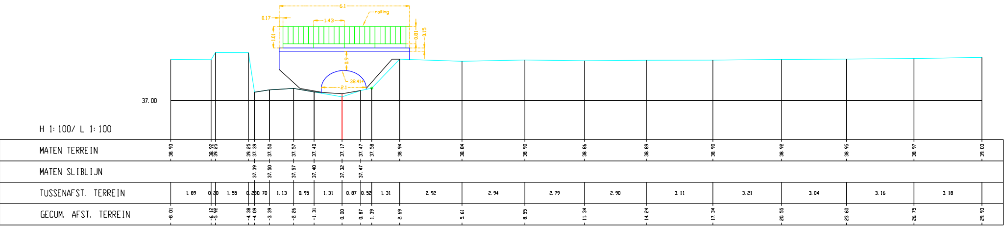
Winge, Dwarsprofiel 479
