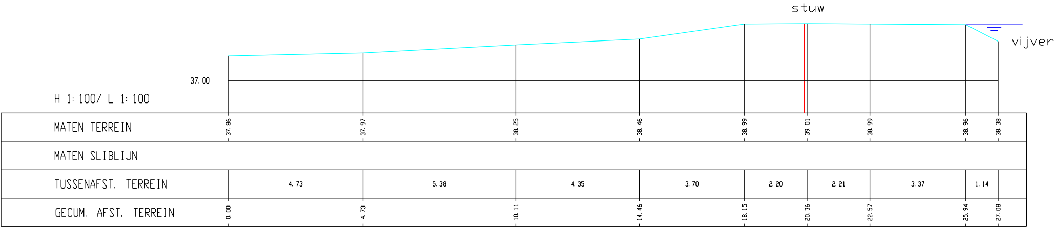
Winge, Dwarsprofiel 487
