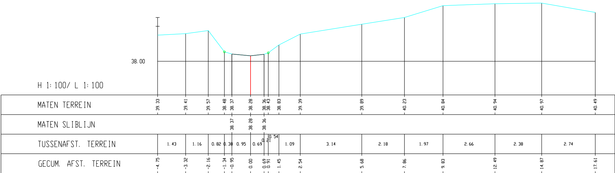
Winge, Dwarsprofiel 490
