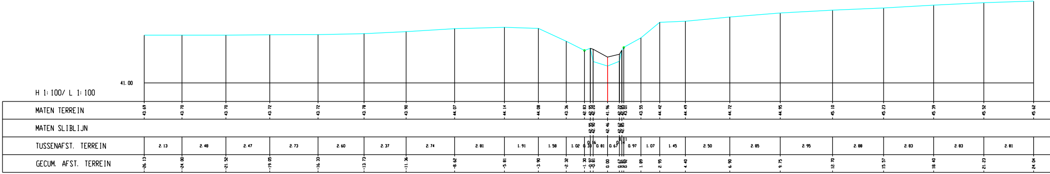
Winge, Dwarsprofiel 539
