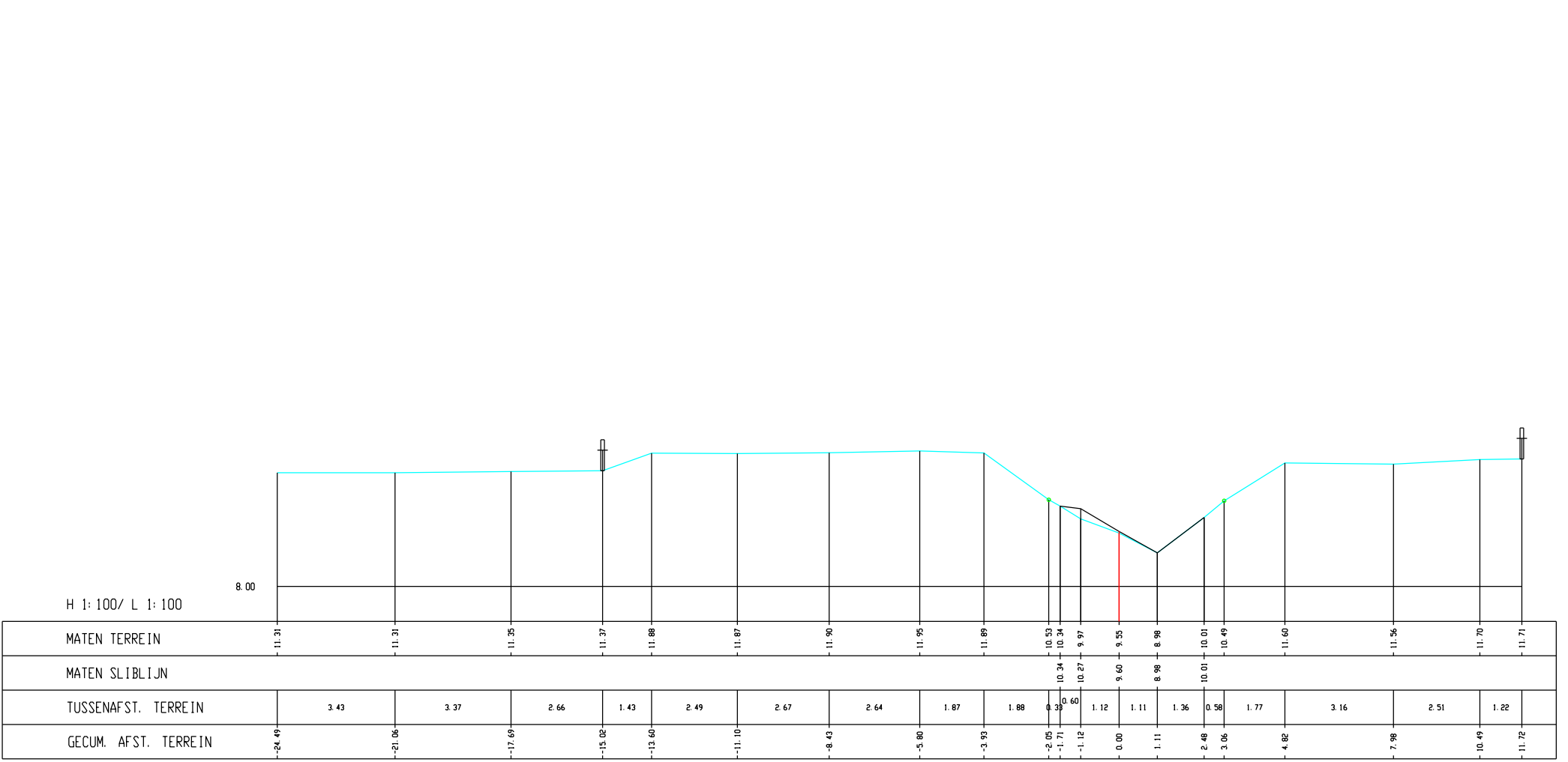
Winge, Dwarsprofiel 058
