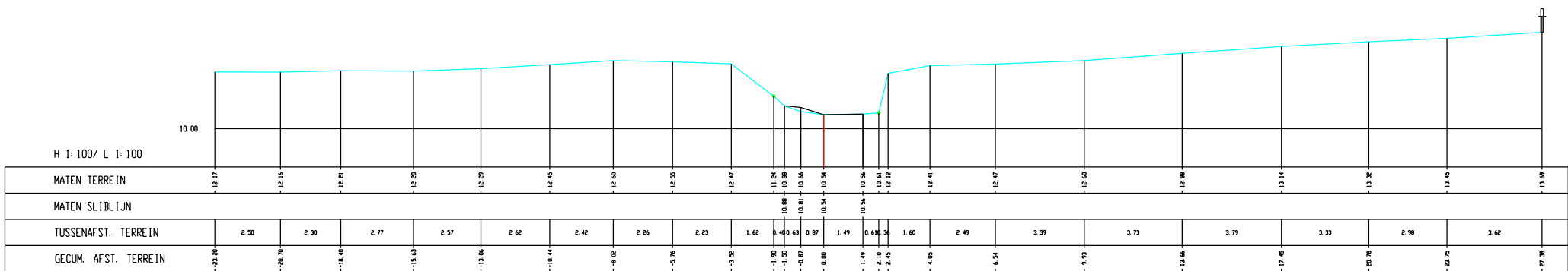
Winge, Dwarsprofiel 084
