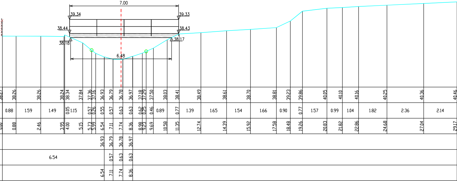
Kunstwerk 6555/401 stroomafwaarts
