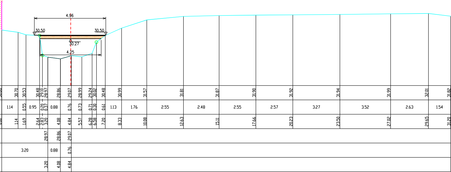
Kunstwerk 6555/191 stroomopwaarts
