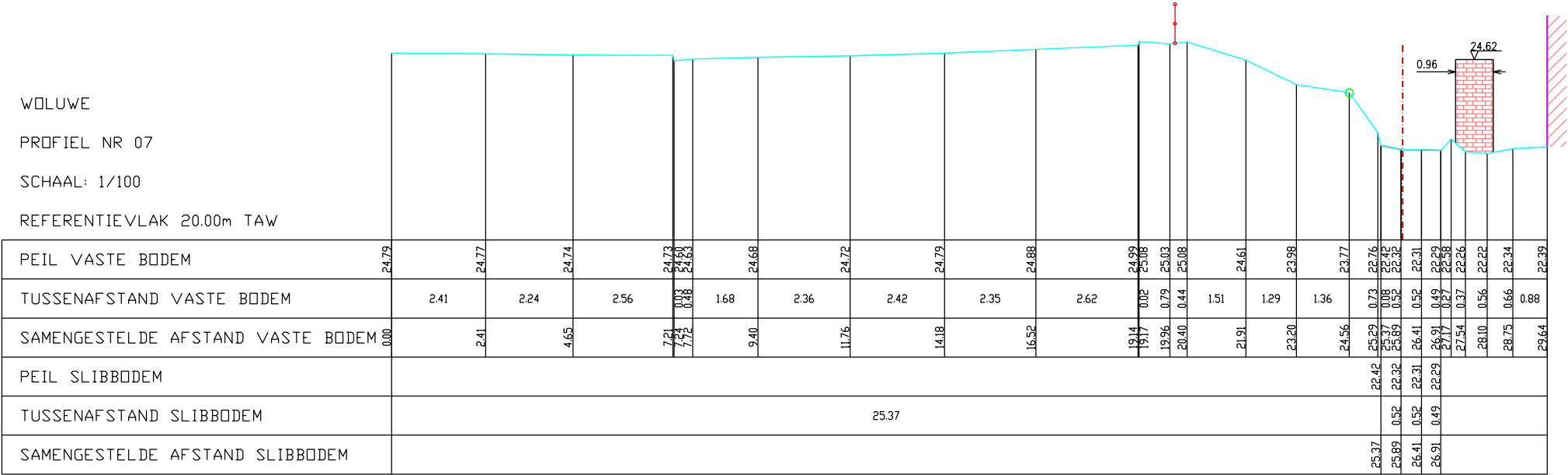
Profiel voor versmalling bij afgebroken watermolen
