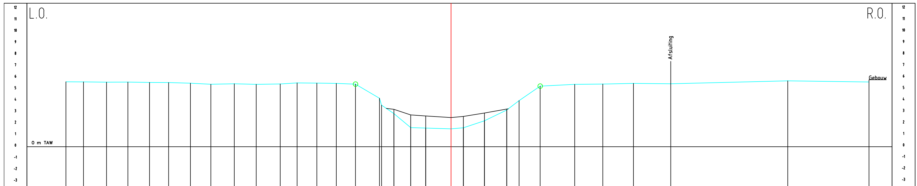
Profiel 266
